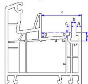
Mitteldichtung
