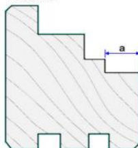
Eurofalz
