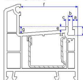
Anschlagdichtung
